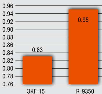
Рисунок 5. Коэффициент готовности гидравлического экскаватора R-9350 (за 3554 моточаса работы) и электрической карьерной мехлопаты ЭКГ-15 (за 18272 моточаса работы)
