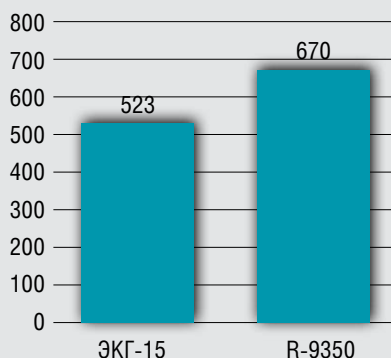
Рисунок 4. Средняя часовая производительность, м³/ч гидравлического экскаватора R-9350 (за 3554 моточаса работы) и электрической карьерной мехлопаты ЭКГ-15 (за 18272 моточаса работы)
