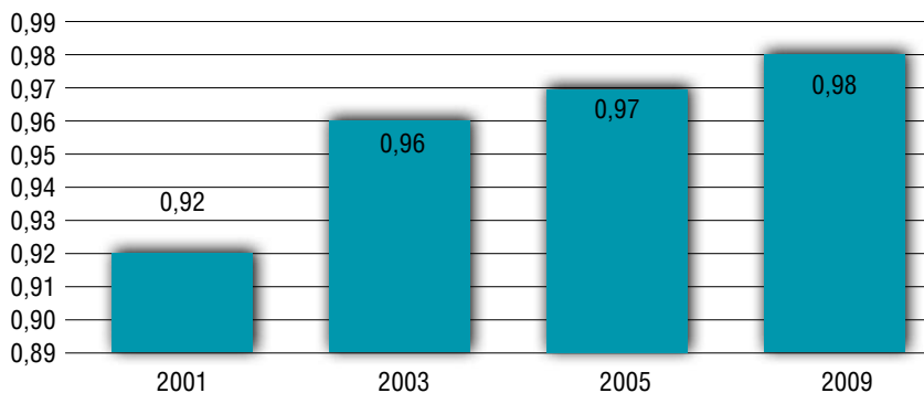
Рисунок 7. Динамика коэффициента готовности экскаваторов по мере освоения технологии обслуживания гидравлических систем в ОАО «Угольная компания «Кузбассразрезуголь»
