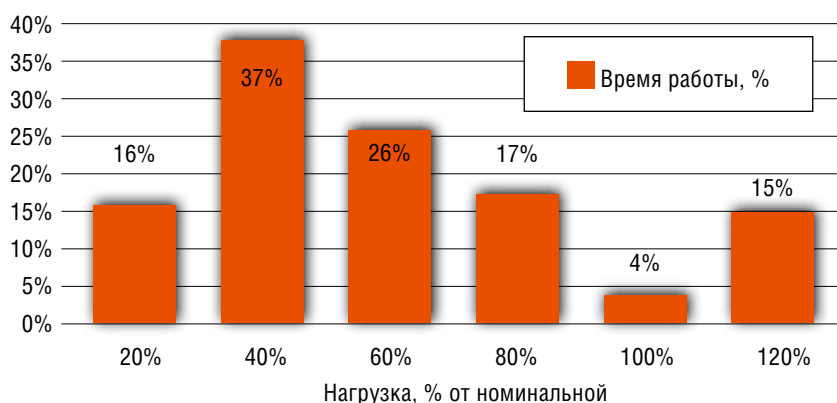
Рисунок 8. Типовая гистограмма нагружения привода карьерного гидравлического экскаватора (по данным непрерывной записи в течение 4500 моточасов)
