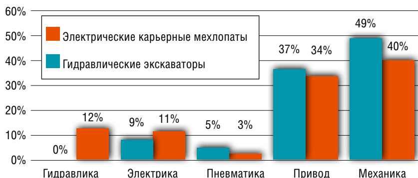
Рисунок 6. Распределение времени аварийных простоев по основным системам электрических карьерных мехлопат и гидравлических экскаваторов, эксплуатируемых в ОАО «Угольная компания «Кузбассразрезуголь»
