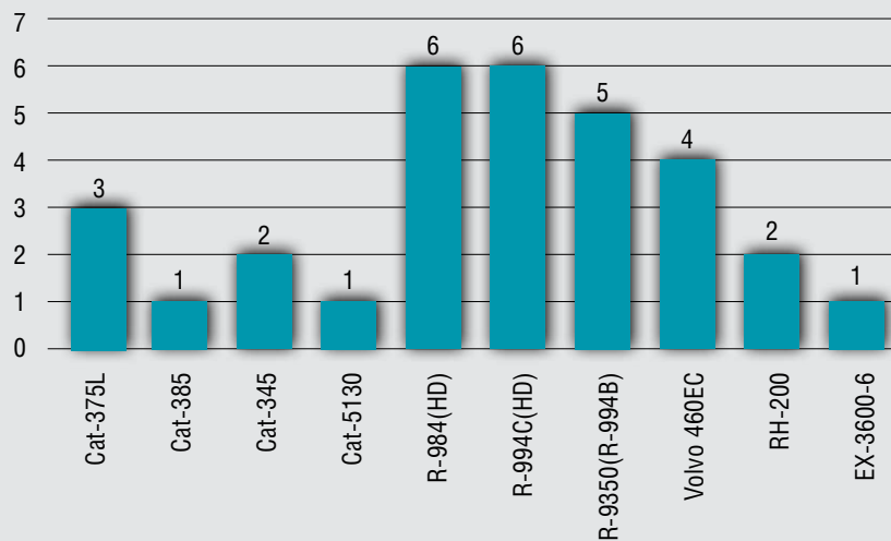
Рисунок 3. Состав парка гидравлических обратных лопат ОАО «Угольная компания «Кузбассразрезуголь» по состоянию на 1 января 2010 года, ед. техники
